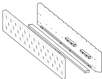
1. Boki x2 + belka środkowa x1
