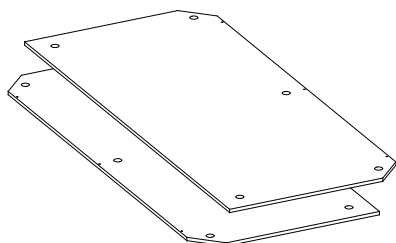
4. Dno pojemnika x2
